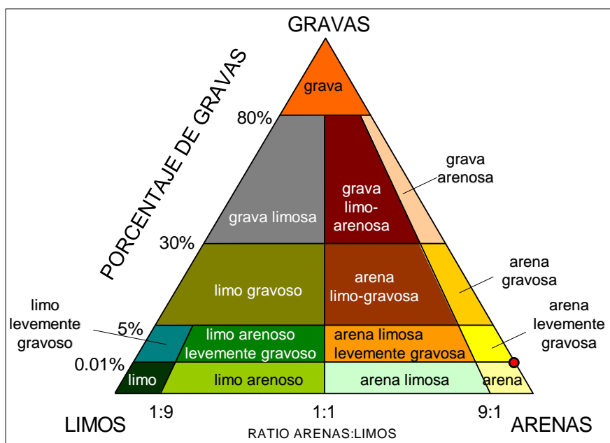
Figura 6.3. Tipo sedimentario según la clasificación de Folk (1974) del sedimento de la estación LEK_SED_01 localizada en Lekeitio (indicado con punto rojo).
